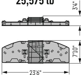
Base plate with erection platform Plaque d'appui avec plateforme de montage
