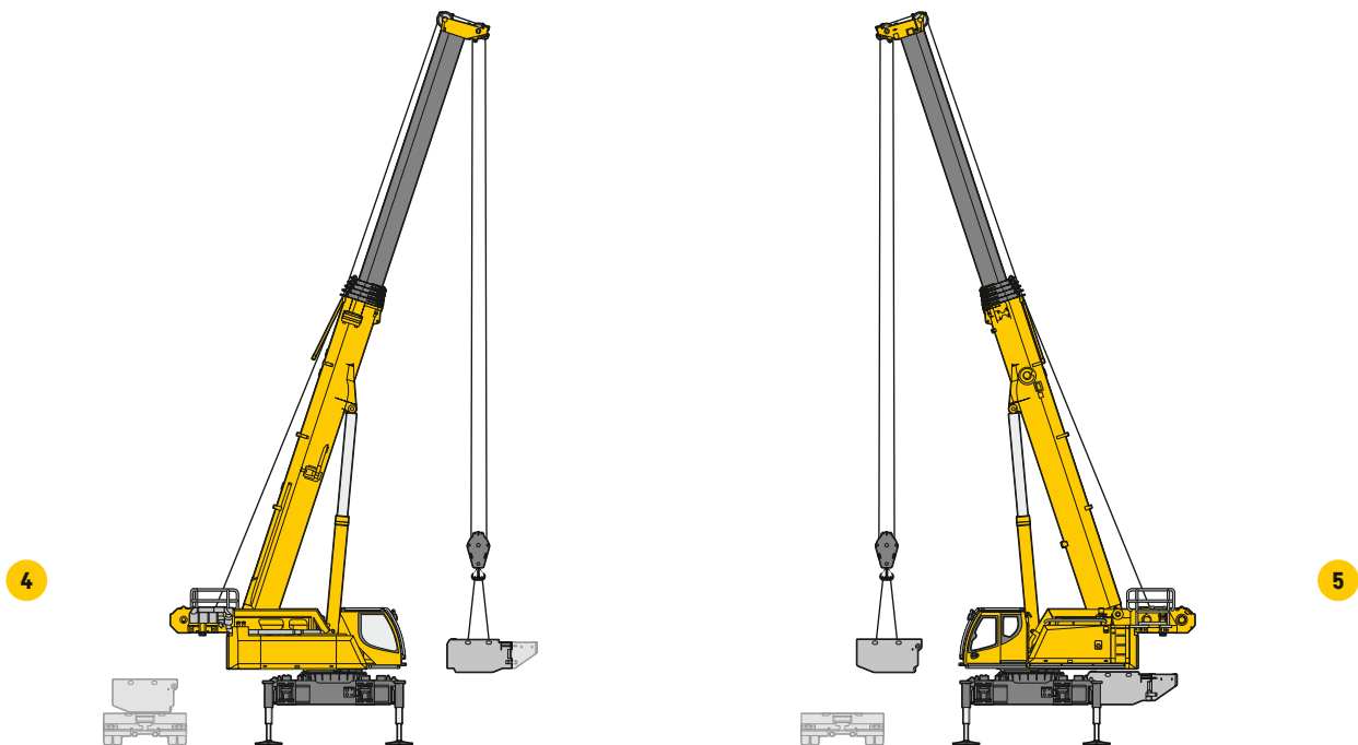
Assemble the central ballast 2x 24,250 lb / Extend the support frame for the superstructure ballast Montage du lest central 2 x 24,250 lb / extension de la réception du lest à plate-forme tournante
